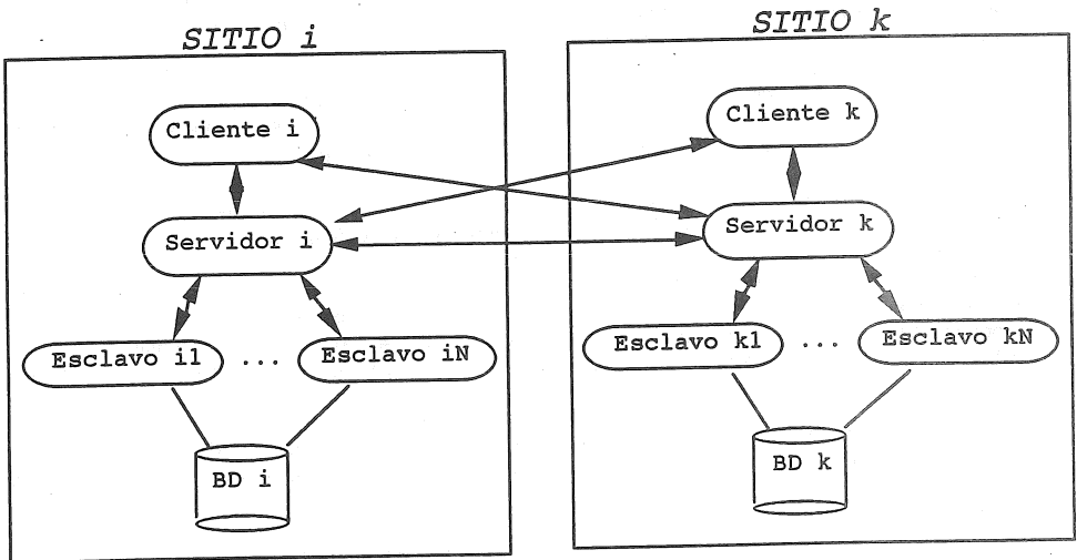
Figura 2. Relación de comunicación entre procesos CLIENTES, SERVIDORES y ESCLAVOS en el sistema PERSEO.
